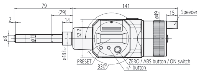
Digitales Anbaumikrometer, Bestell-Nr. 00-99-901-4889
