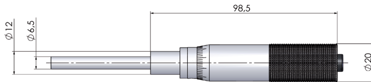
Analoges Anbaumikrometer, beispielhafte Darstellung Bestell-Nr. 00-30-000-6804
